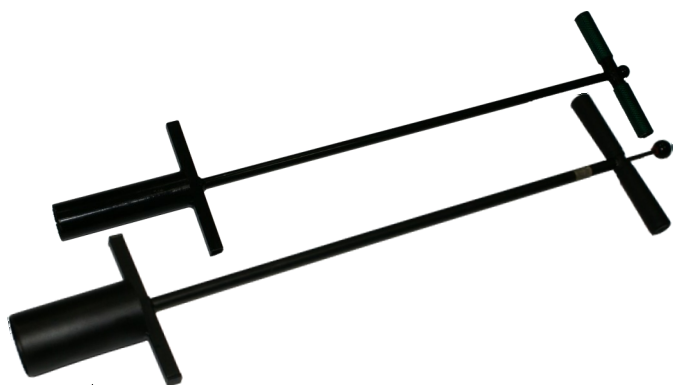
▲ Kosztury (dołowniki) do wysadzania
